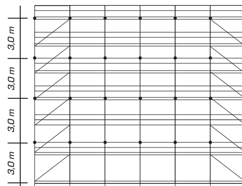
Afstand forankringsrør 3,0 m Maks. søjlelast 20,5 kN
