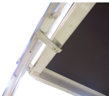
Pat. stormlås til sikring af dæk. Passer til alle typer stillads
